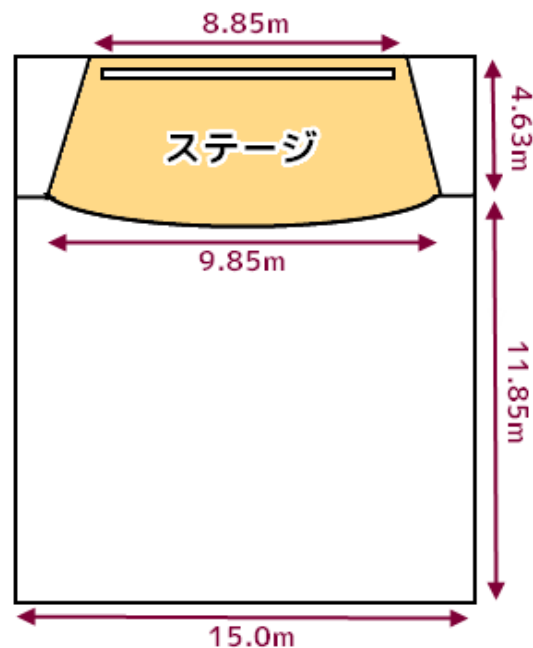
◆マルチメディアホール簡易見取り図
